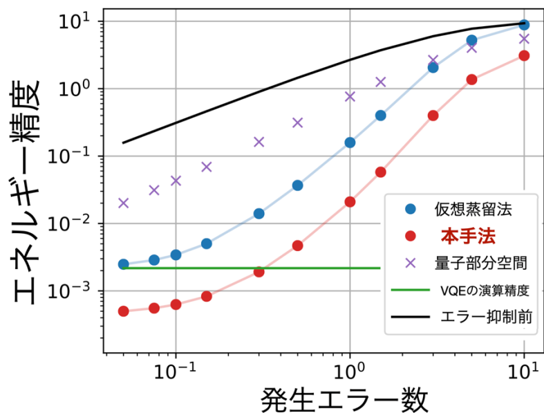
図3：変分量子アルゴリズムの一種である、変分量子固有値ソルバ（VQE）による演算自体が不完全、かつ量子コンピュータ上にノイズが発生した場合の計算精度。発生エラー数が1程度以下の場合には、計算されるエネルギー精度が大きく異なる。つまり、エラー抑制手法による性能差が顕著に現れることが読み取れる。特に本手法を用いた場合には、VQE自体の演算よりも精度の良い計算が可能となる。すなわち、VQEに内在する誤差も抑制することができる。これは、仮想蒸留法や量子部分空間展開法といった従来手法では達成できない領域である。
