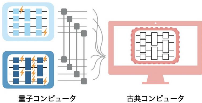
図 1：ノイズの強さが異なる複数の量子状態を用いた量子多体計算の概念図。本研究で提案された手法では、複数の状態を干渉させた結果の適切な組み合わせ方法を、古典コンピュータ上で補助的に計算した上で、最終的な計算結果を出力する。
